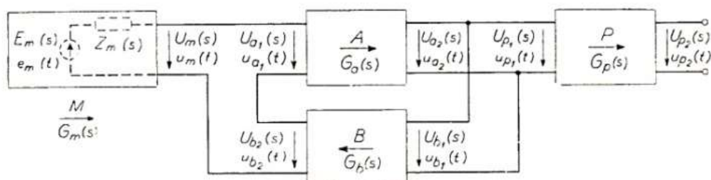
Fig. 3.1 Blockschema över ett automatiskt regleringssystem. M ordregivningselement; A regleringselement; B återkopplingsselement; P indirekt reglerat system.
